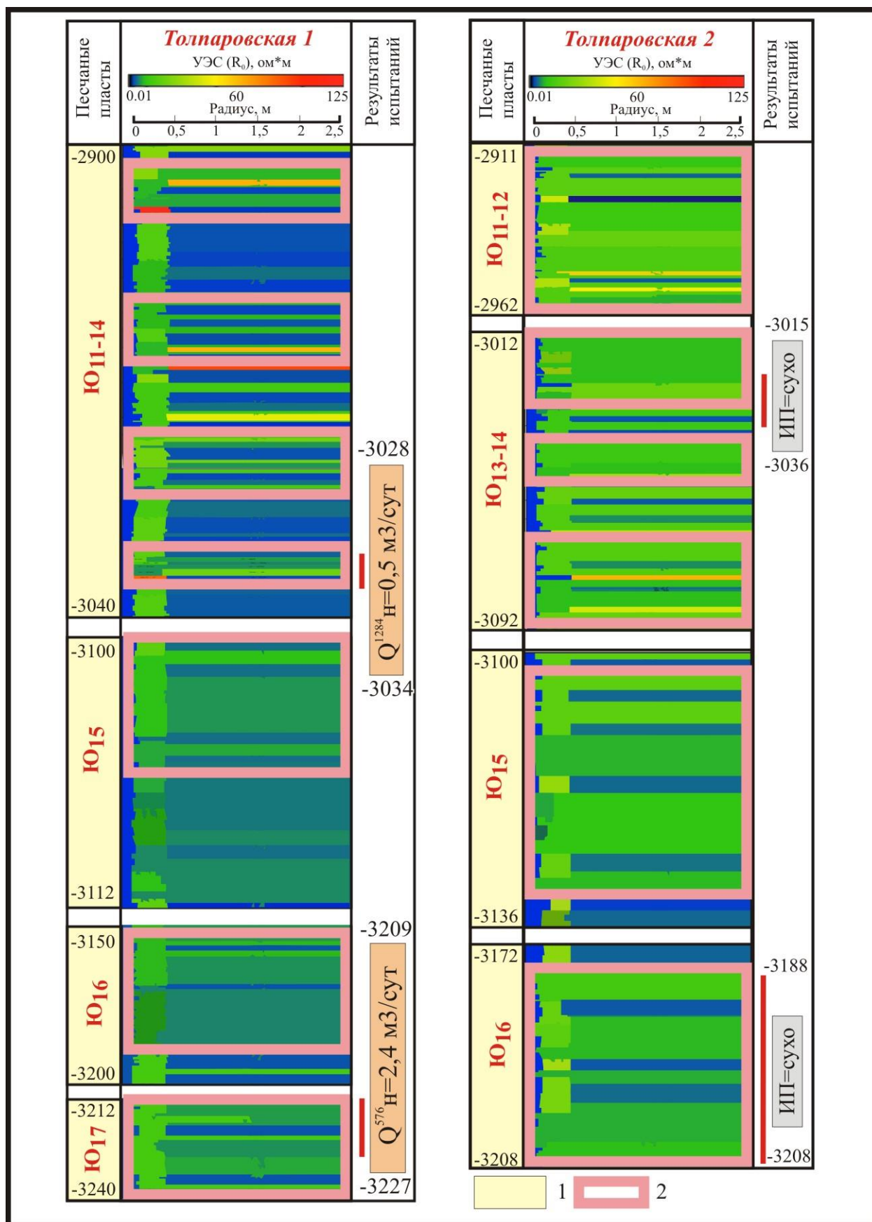
Рисунок 5.20 – Результаты интерпретации данных БКЗ в коллекторах геттанг-ааленских отложений на основании одномерной численной инверсии в скв. Толпаровские № 1 и № 2.
