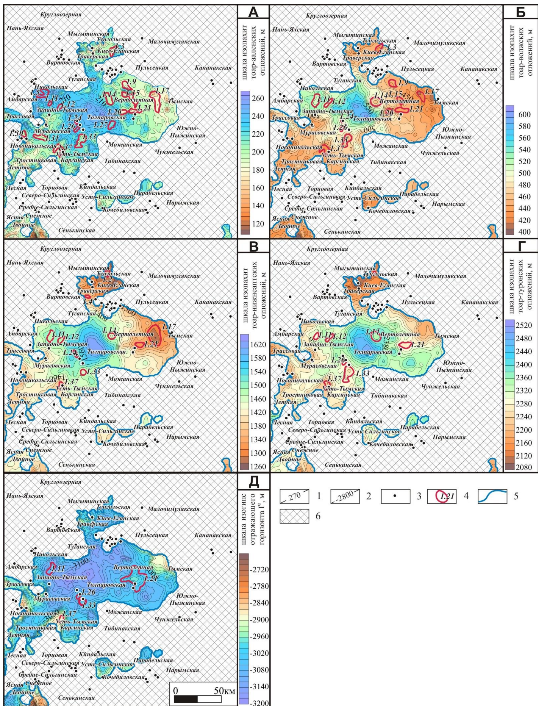
Рисунок 3.7 - Динамика изменения рельефа кровли урманской свиты на время формирования нижнетюменской подсвиты (горизонт I^a ) (аален) (А), баженовской свиты (горизонт II^a ) (волга) (Б), кошайской пачки алымской свиты (III) (апт) (В), кузнецовской свиты (IV) (турон) (Г); современный рельеф (Д).
