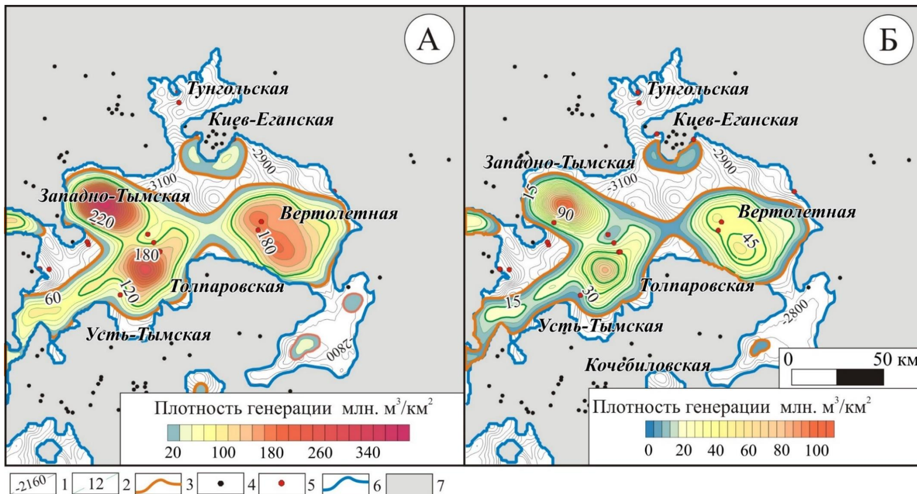
Рисунок 5.7 - Карты современных кумулятивных масштабов генерации газообразных УВ органическим веществом тогурской свиты для II (А) и III (Б) типов керогена в Усть-Тымском очаге.
