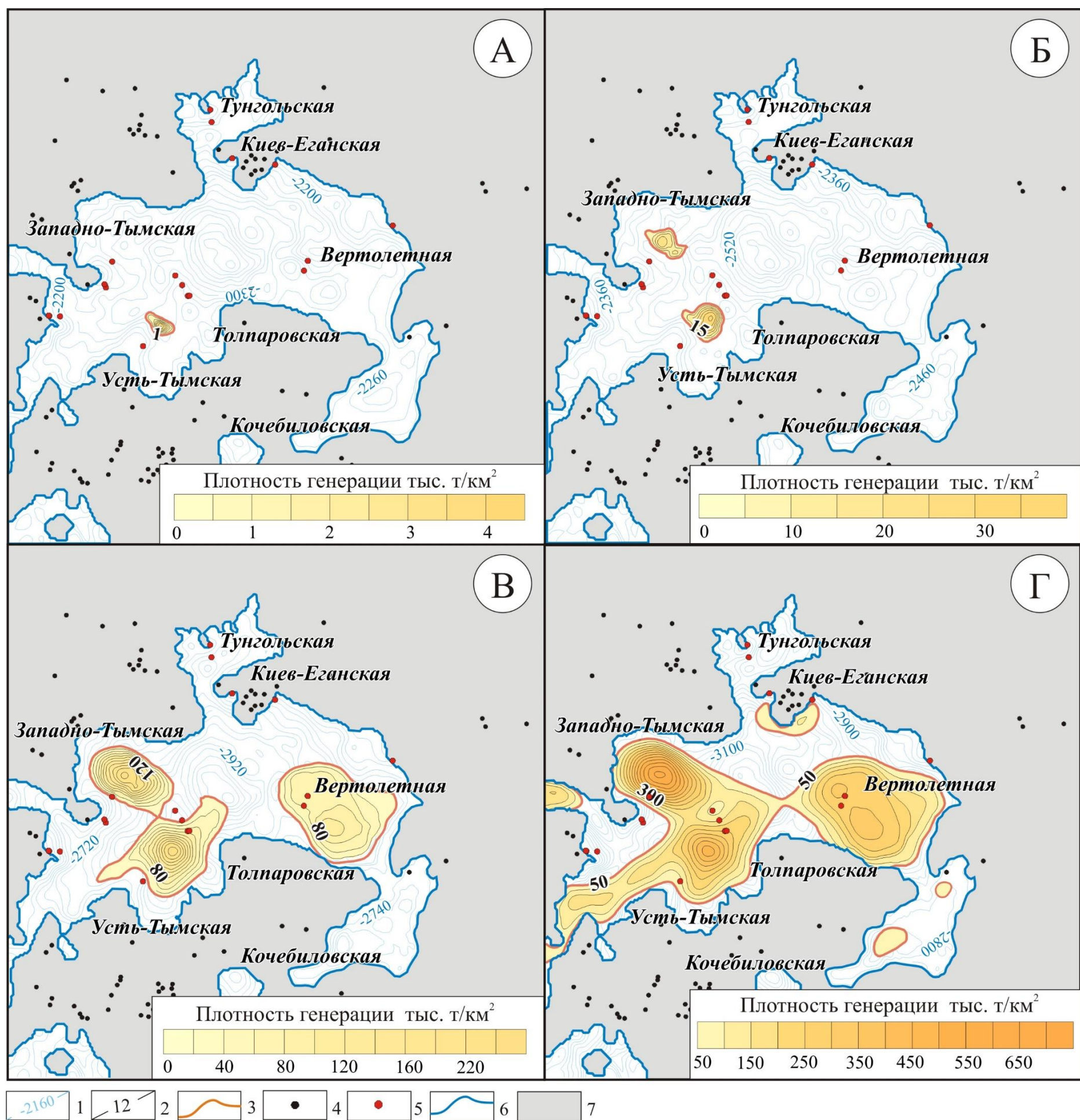
Рисунок 5.6 – Карты кумулятивных масштабов генерации жидких УВ органическим веществом тогурской свиты для III типа керогена в Усть-Тымском очаге на время формирования свит: А - кузнецовской (89.8 млн лет), Б - ипатьевской (83.6 млн лет), В - талицкой (61.6 млн лет); Г – на настоящее время.
