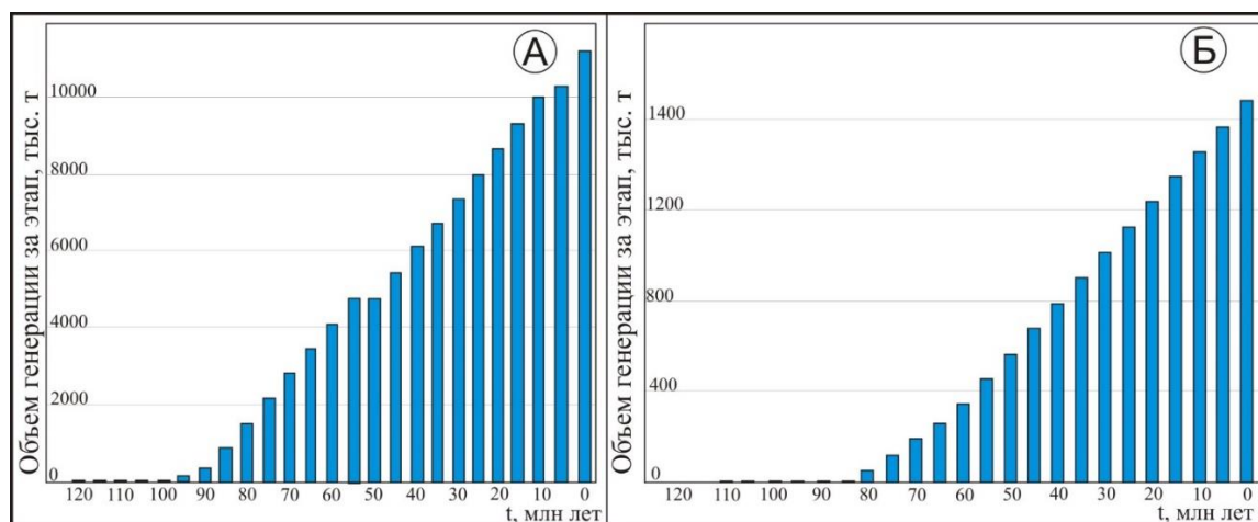
Рисунок 5.8 - Диаграммы генерации жидких УВ органическим веществом тогурской свиты для керогена II типа (А) и керогена III типа (Б) во времени.
