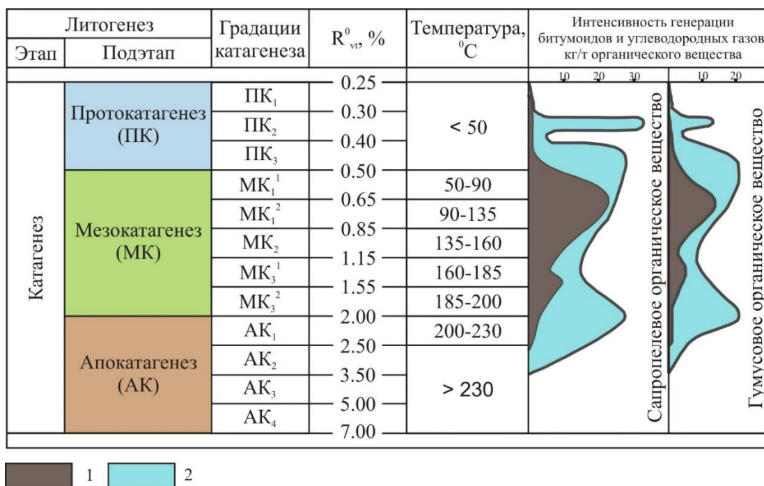
Рисунок 5.2 – Интенсивность образования нефти и газа [Конторович, Трофимук, 1976].
