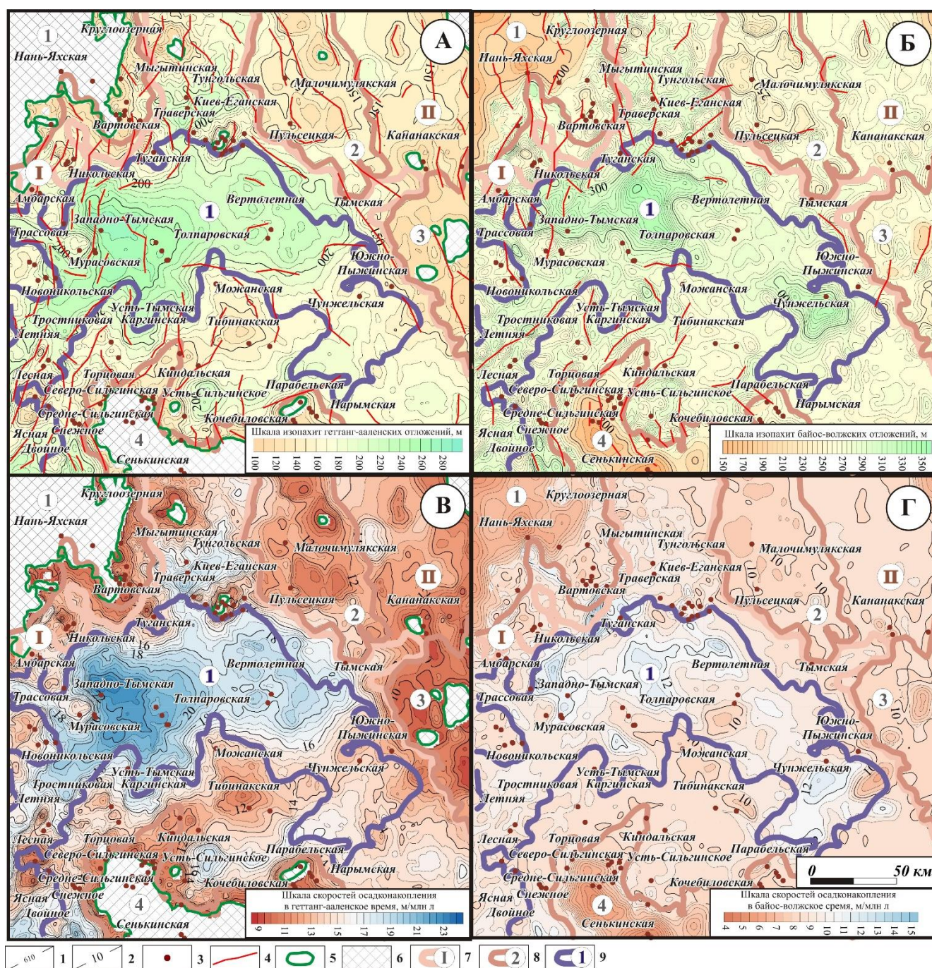
Рисунок 3.3 – Карты скоростей осадконакопления в геттанг-ааленское (А) и байос-волжское (Б) время и карты толщин сейсмогеологических комплексов: В – геттанг-ааленского, Г – байос-волжского.
