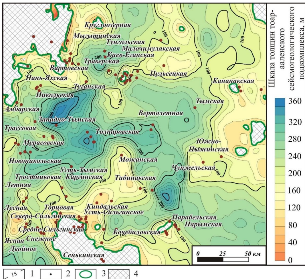
Рисунок 4.7 – Карта толщин тоар-ааленского сейсмогеологического подкомплекса.
