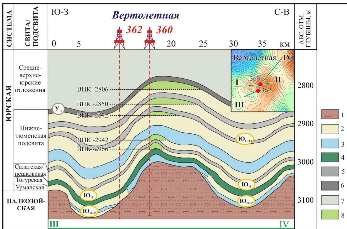
Рисунок 5.30 - Геологический разрез геттанг-ааленских отложений на Вертолетной площади по линии III-IV (см. Рисунок 5.22).
