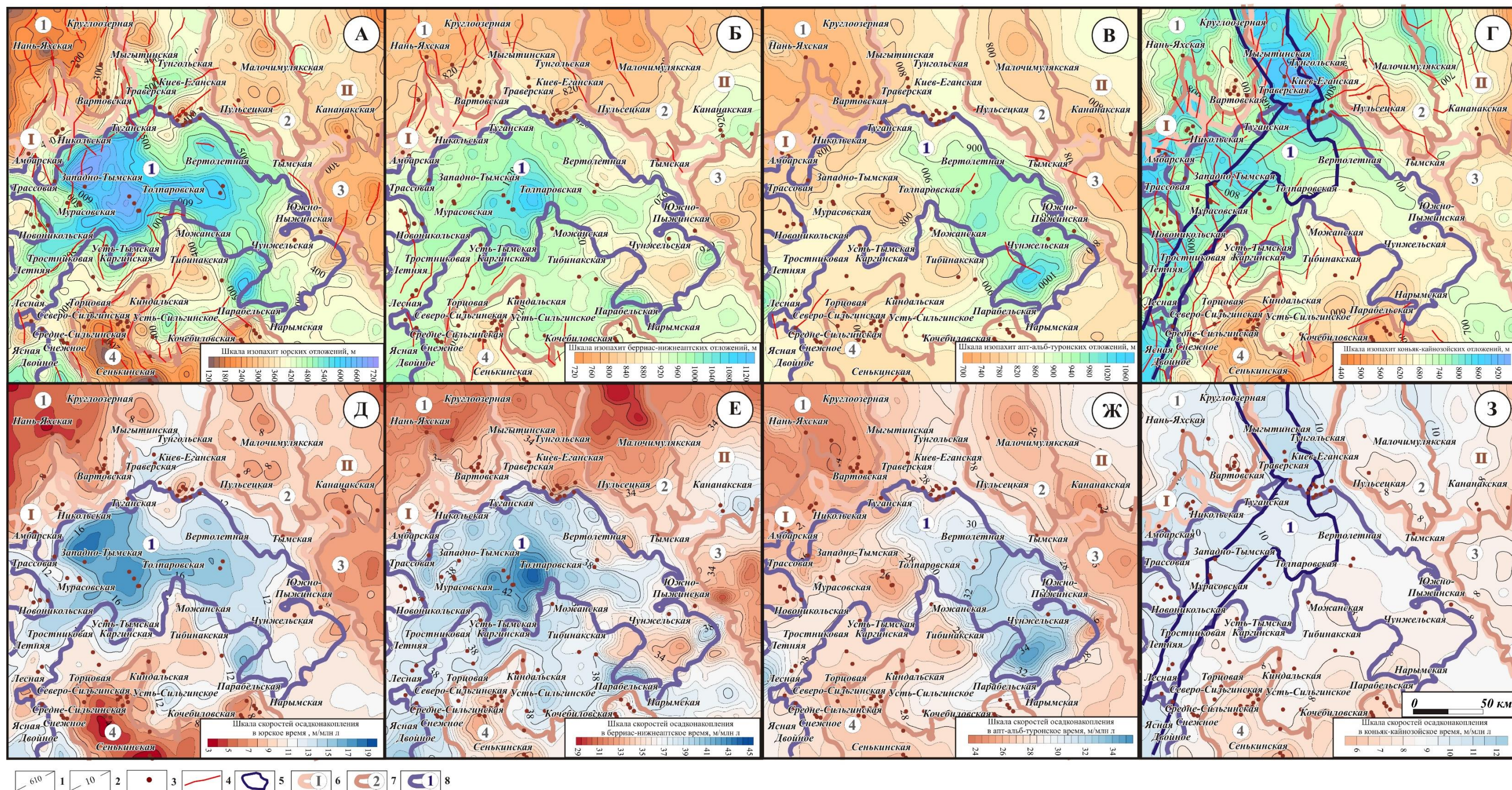
Рисунок 3.4 – Карты толщин и скоростей осадконакопления сейсмогеологических комплексов/мегакомплексов: юрского (А, Д), берриас-нижеаптского (Б, Е), апт-нижнетуронского (В, Ж), коньяк-кайнозойского (Г, З).
