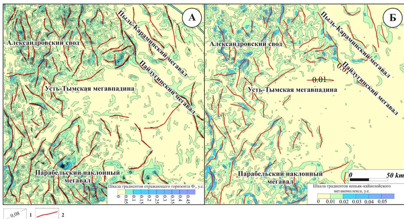
Рисунок 2.4 – Выделение разрывных нарушений на картах градиентов по структурной поверхности кровли доюрского основания (Ф 2 ) (А) и по карте изопахит коньяк-кайнозойского мегакомплекса (Б).
