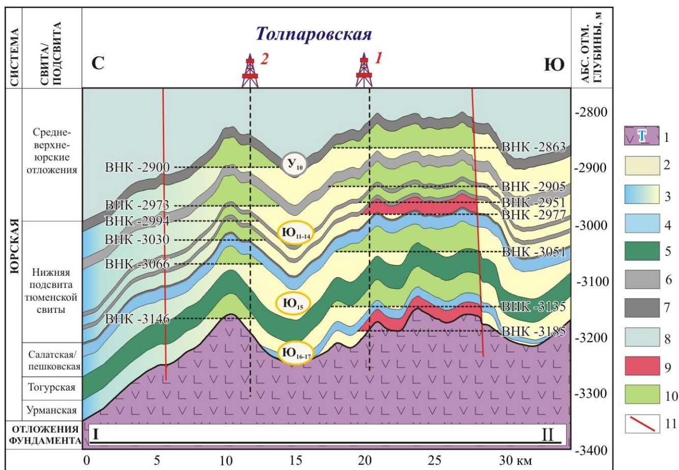
Рисунок 5.22 - Геологический разрез геттанг-ааленских отложений на Толпаровской площади по линии I-II (см. Рисунок 5.21).
