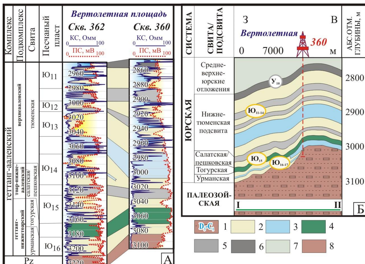
Рисунок 5.27 – Корреляционная схема геттанг-ааленских отложений Вертолетной площади (А) и геологический разрез (Б).
