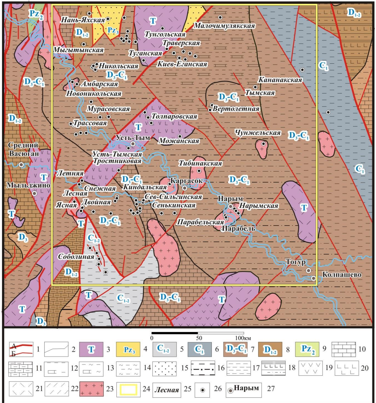
Рисунок 1.3 - Карта вещественного состава пород доюрского основания [Обобщение результатов..., 2007 ф].
