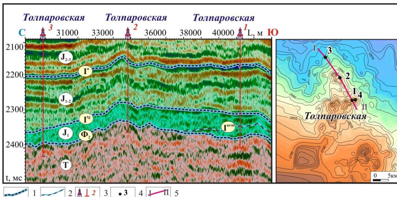
Рисунок 5.15 – Фрагмент временного разреза, пересекающего Толпаровскую площадь.
