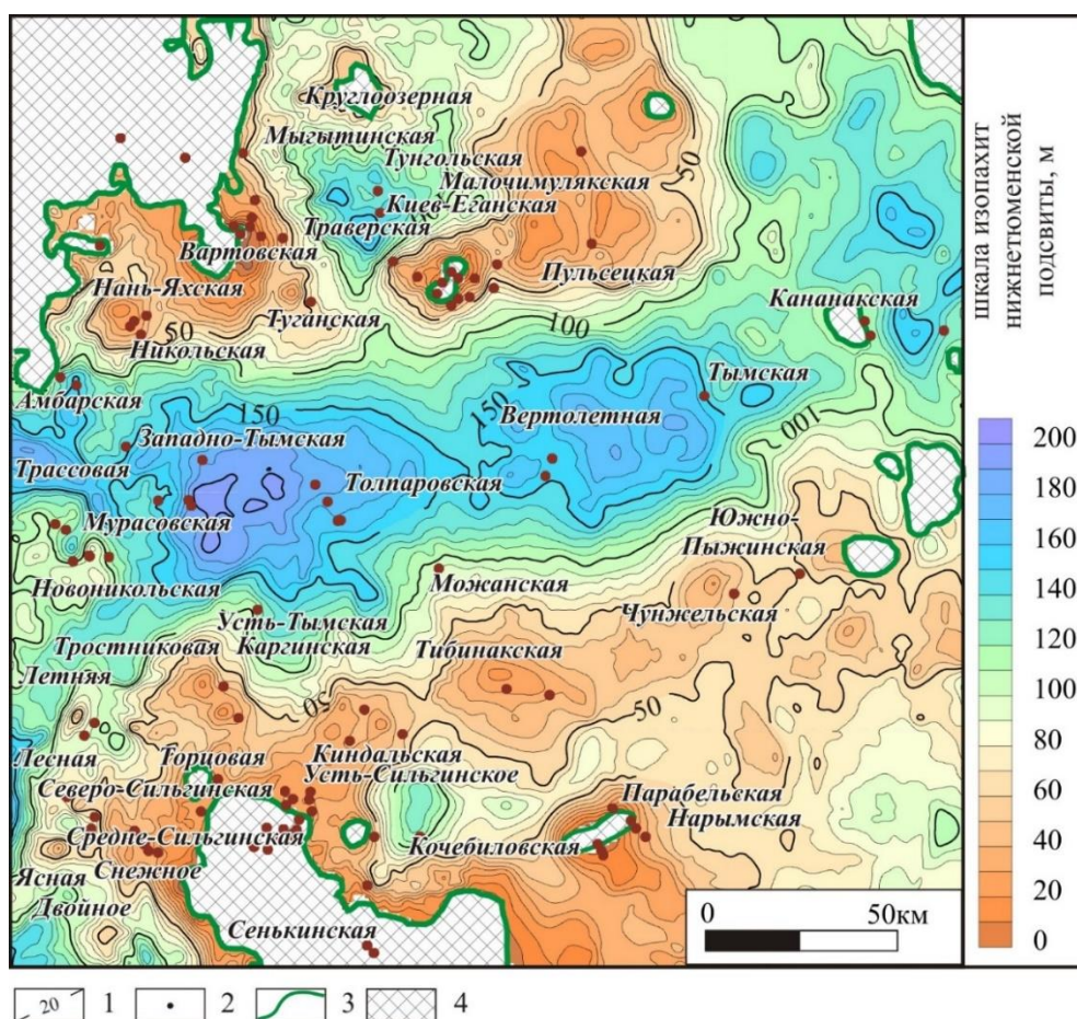
Рисунок 4.9 - Карта толщин нижней подсвиты тюменской свиты.
