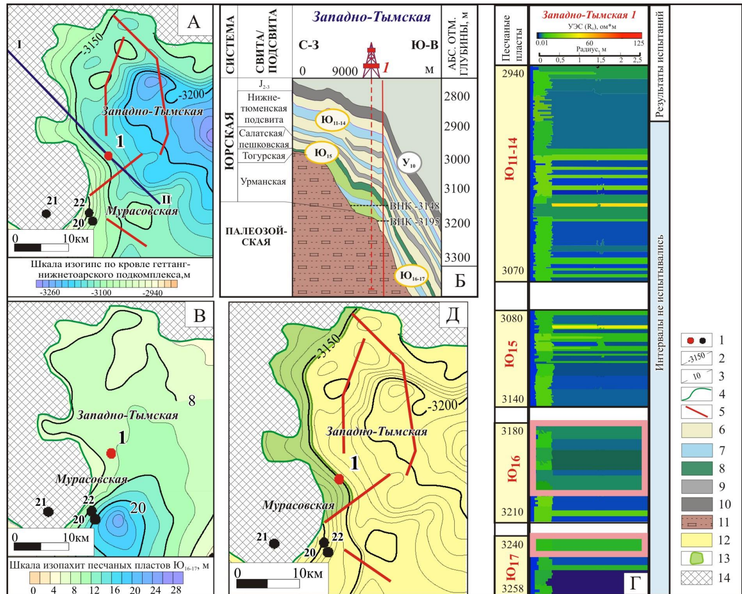
Рисунок 5.25 – Характеристика Западно-Тымской площади: А – структурная карта по кровле геттанг-нижнетоарского подкомплекса, Б – геологический разрез по линии I-II, В – карта эффективных толщин геттанг-нижнетоарского подкомплекса, Г – модель БКЗ скв. Западно-Тымская № 1, Д – карта распределения перспективных объектов.
